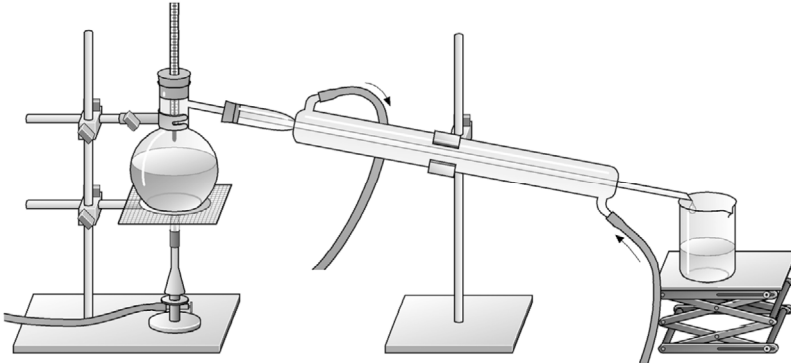
Destillieren
