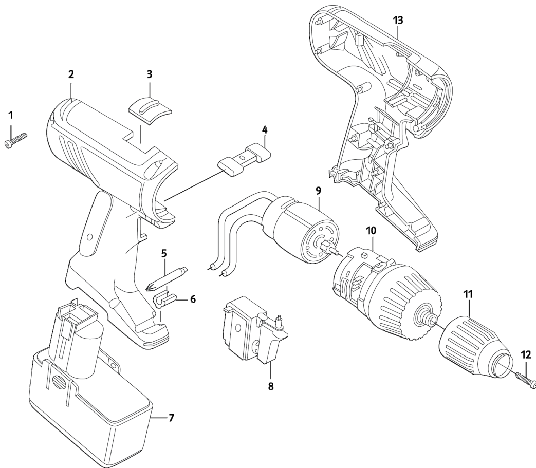
1 Explosionszeichnung eines Akku-Bohrschraubers
